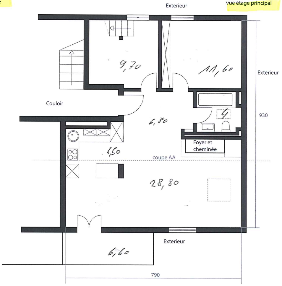
coupe AA
